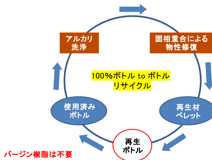
図 6 再生材 100%使用の PET のボトル to ボトル技術
