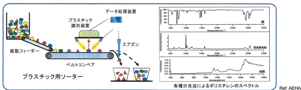
図 10 プラスチックの高度選別技術
