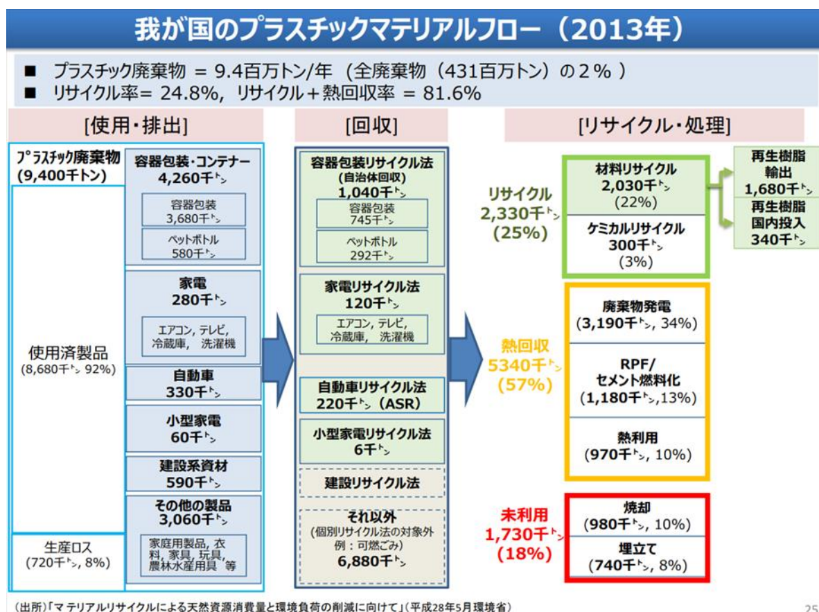
図3 我が国のプラスチックマテリアルフロー図(2013年)
