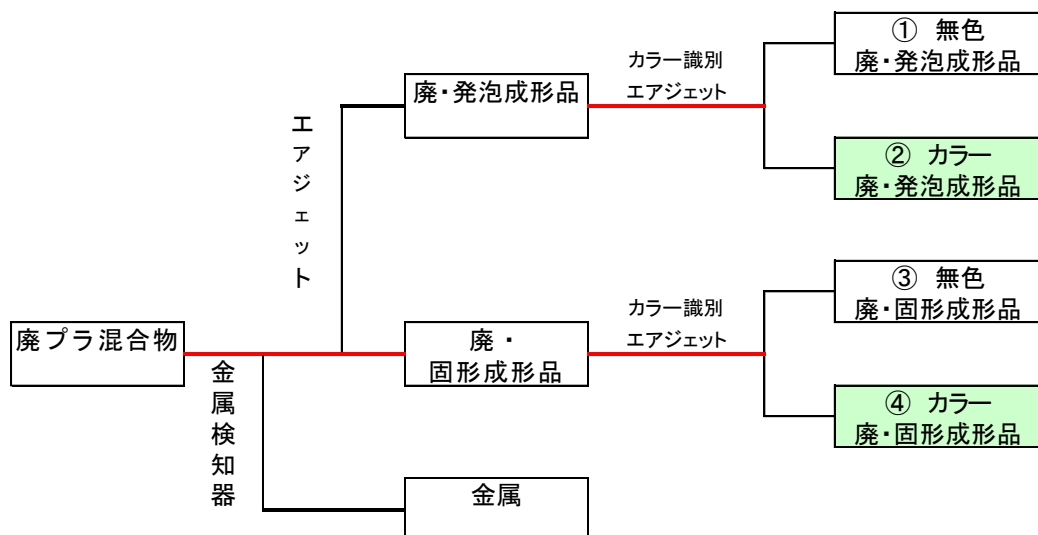
図 11 選別の第 1 スキーム(発泡体と固形物の選別と無色透明物とカラー着色物の選別)
