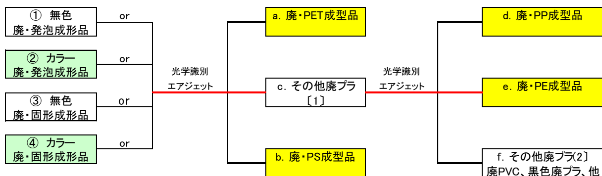
図 12 選別の第 2 スキーム(材質別分別)
